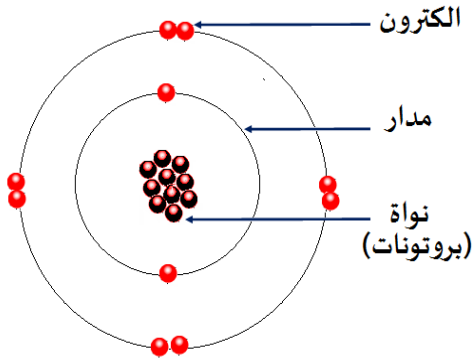
نموذج الذرة
